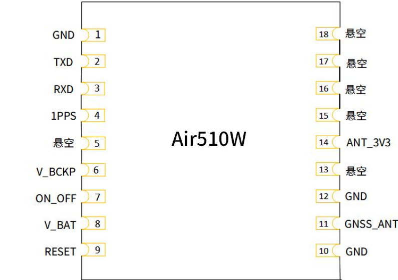
模块管脚示意图:
