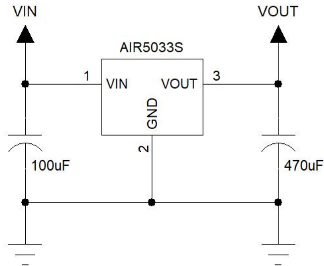
图 6: Air5033S 供电输入参考设计
