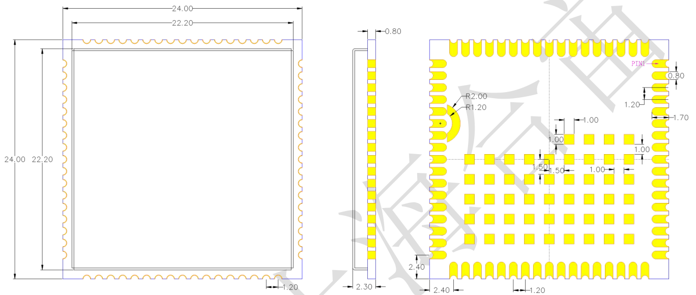
图表 22: Air724UG 尺寸图 (单位: 毫米)
