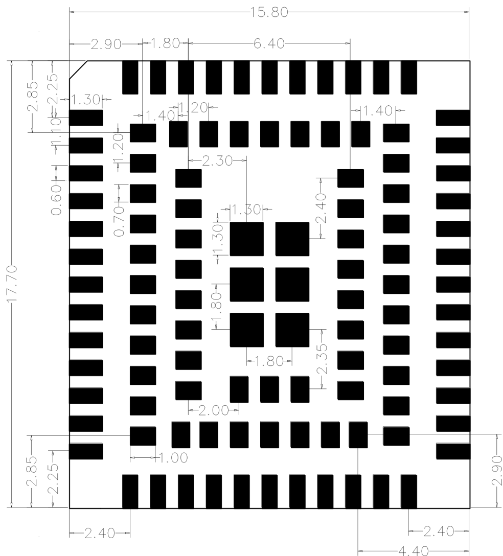
正视图，Air780EG PCB 封装（单位：毫米）
