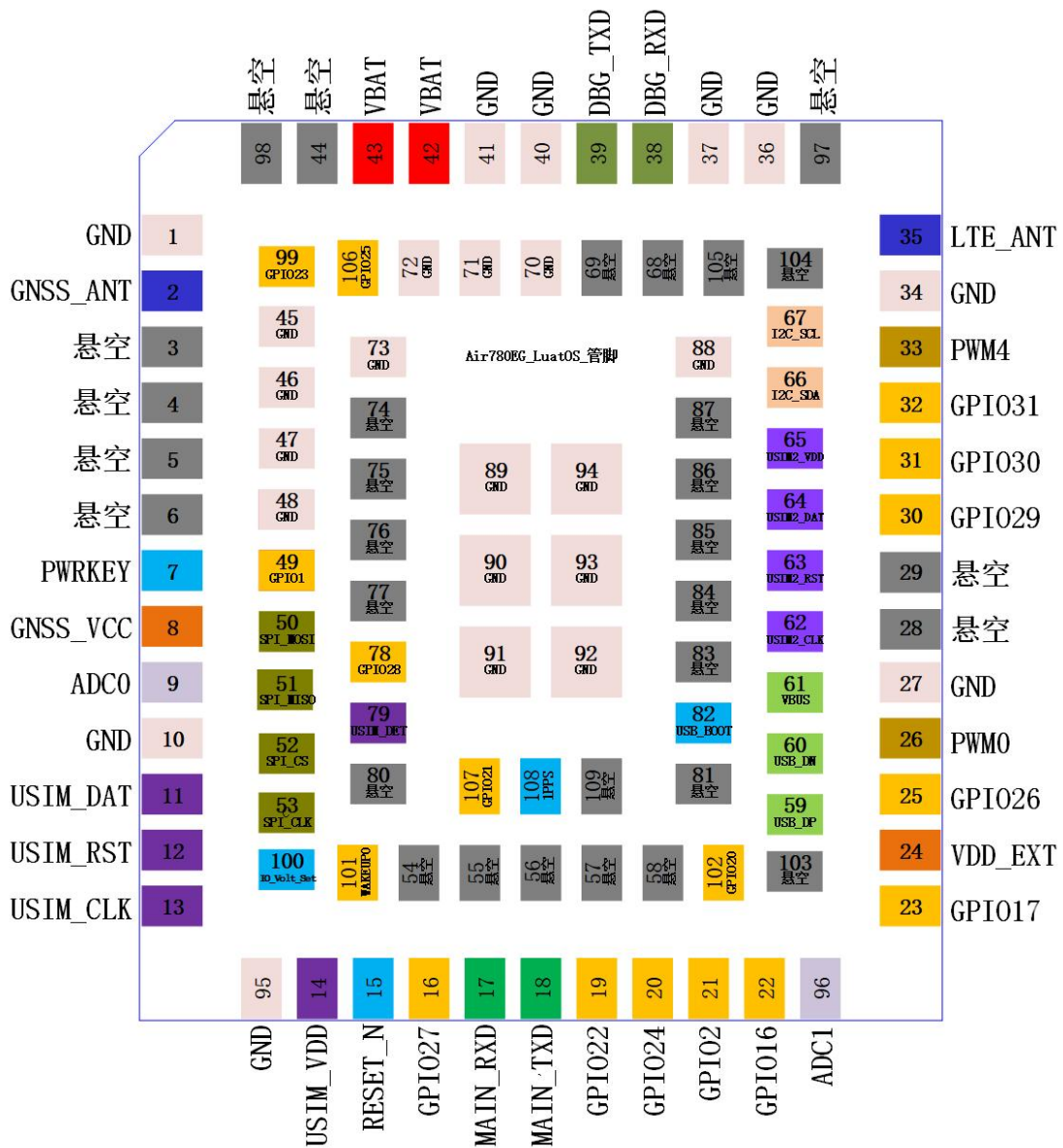
管脚透视图
