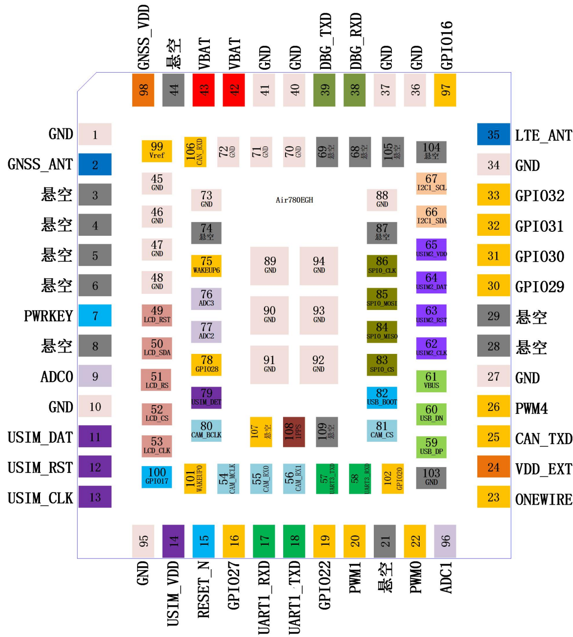
管脚透视图
