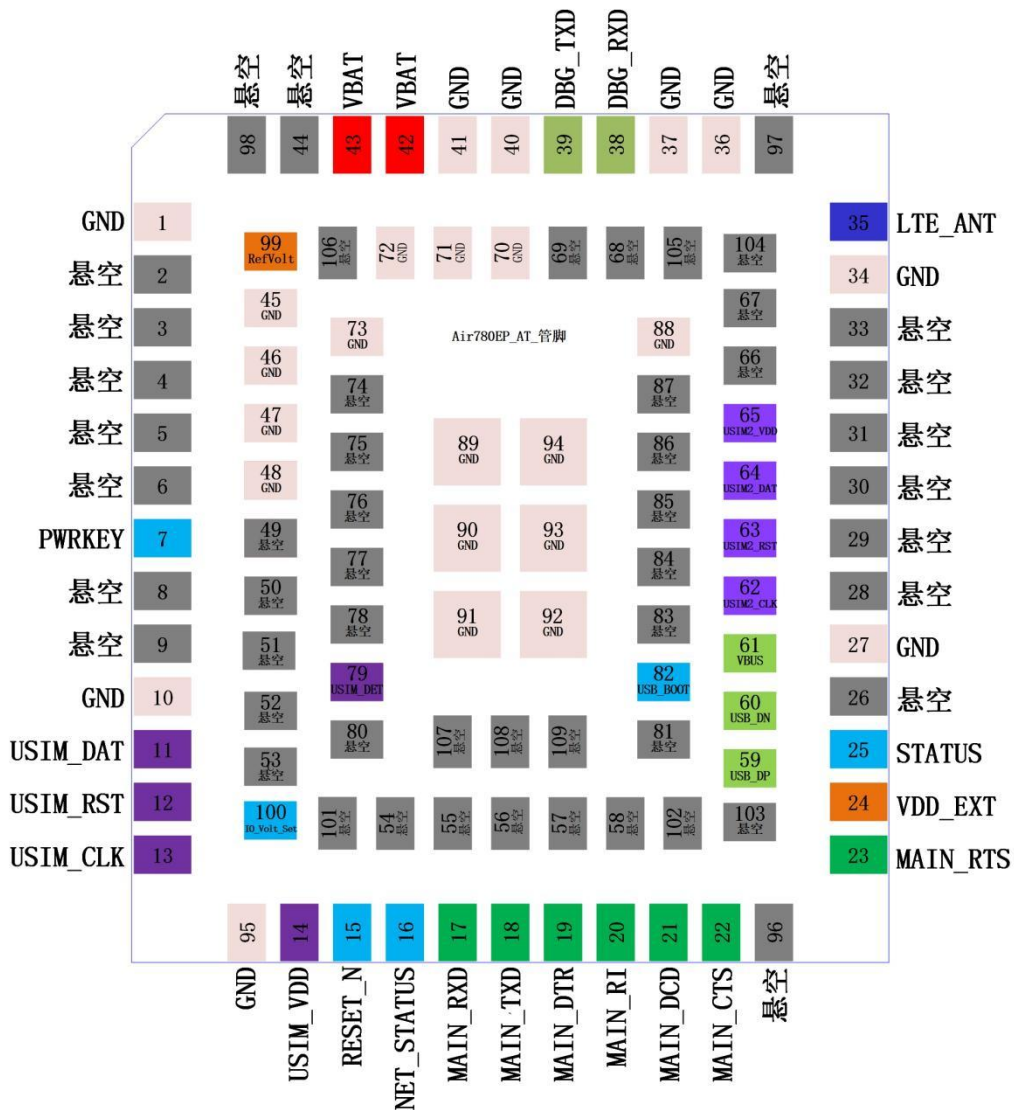
管脚透视图
