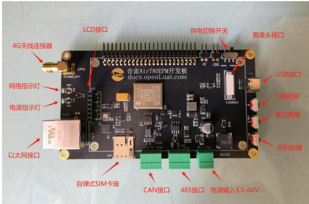
顶视图
