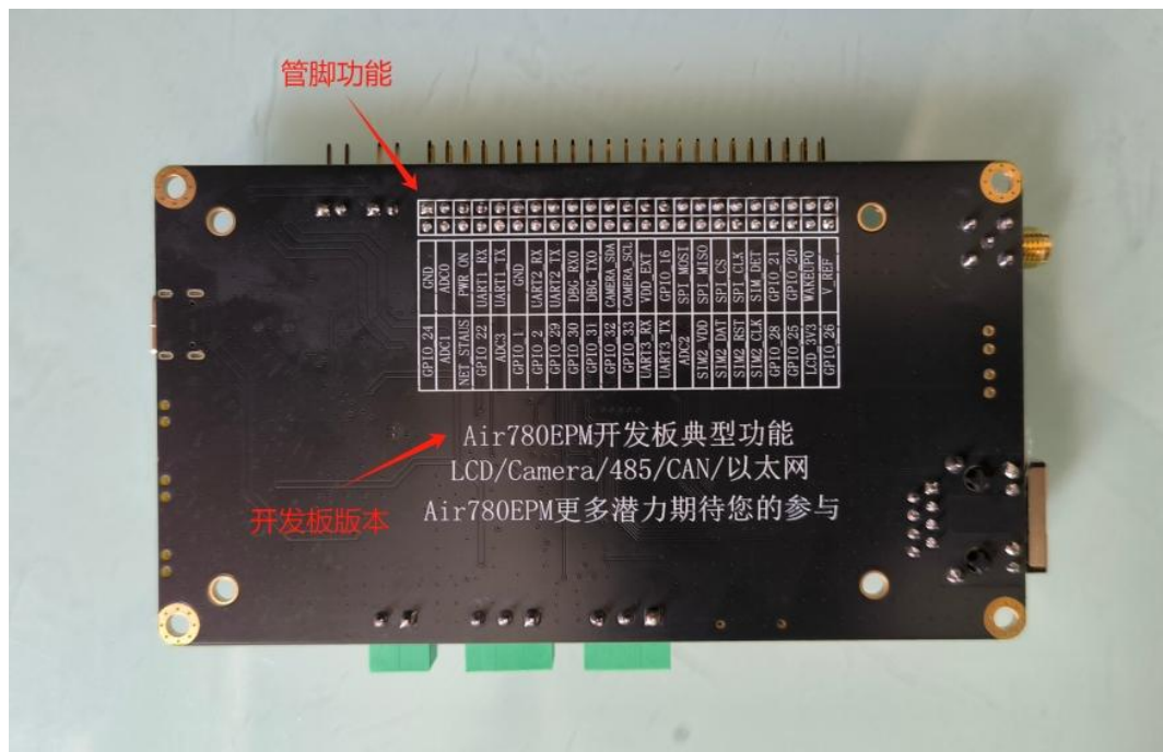
底视图
