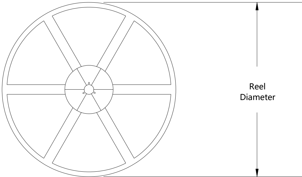
Reel Dimensions
