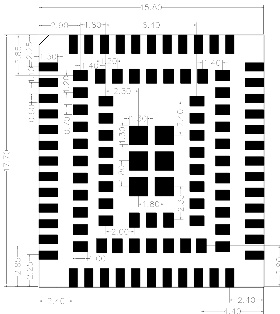
正视图，Air780EQ PCB 封装（单位：毫米）
