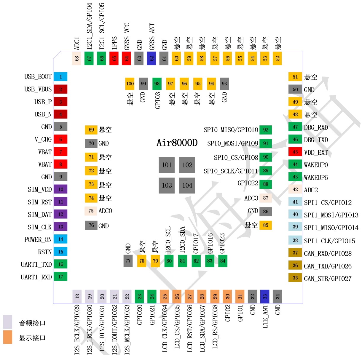
图 5: Air8000D 管脚排列图 (正视图)
