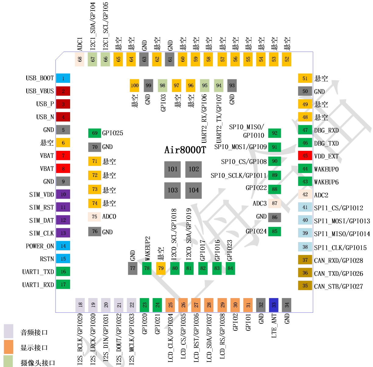
图表 6: Air8000T 管脚排列图 (正视图)
