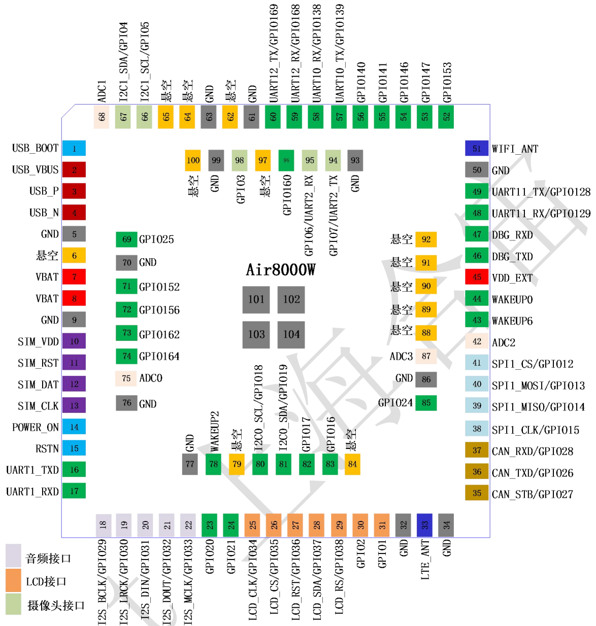
图 3: Air8000W 管脚排列图（正视图）
