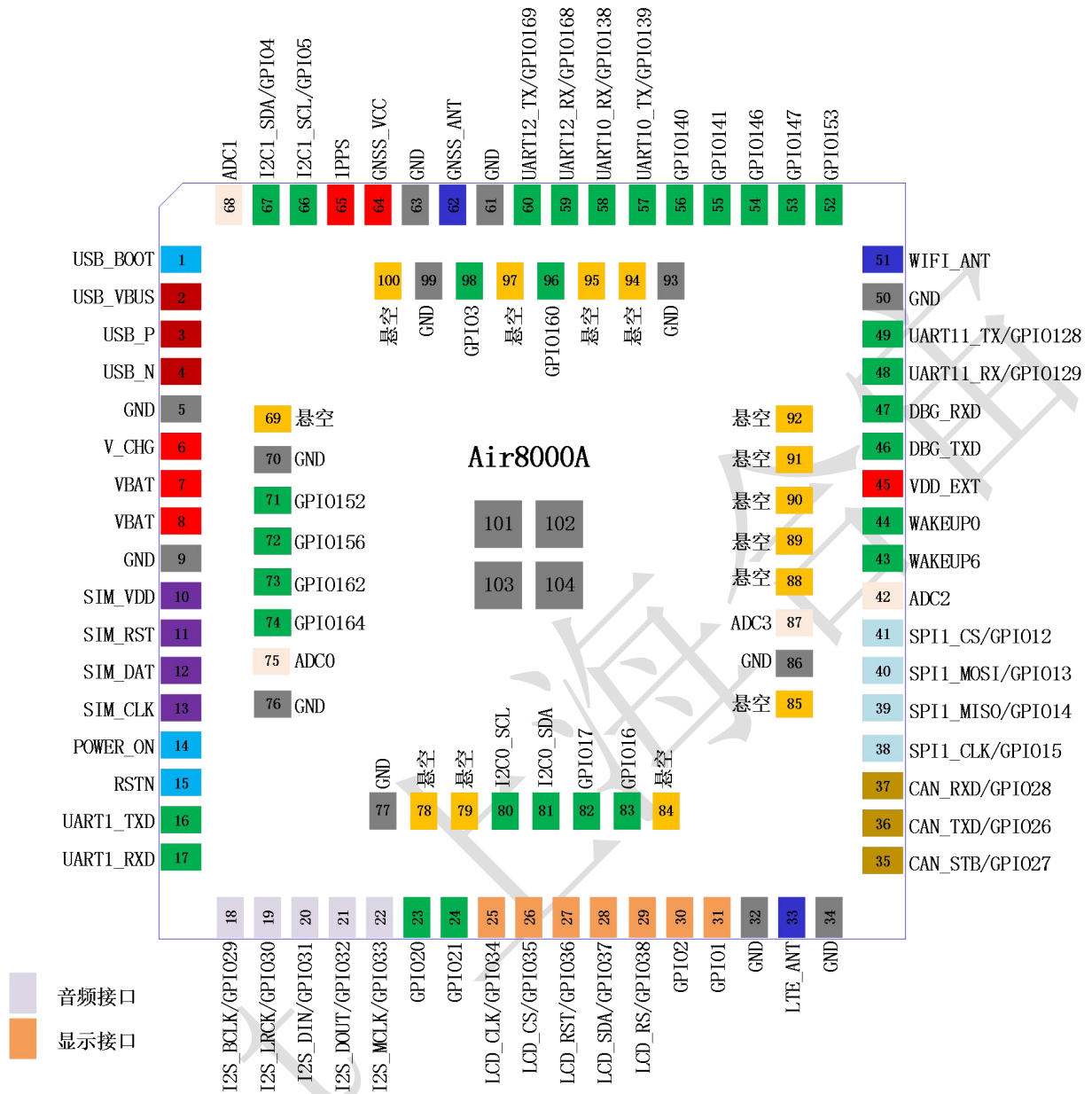
图表 3：Air8000A 管脚排列图（正视图）
