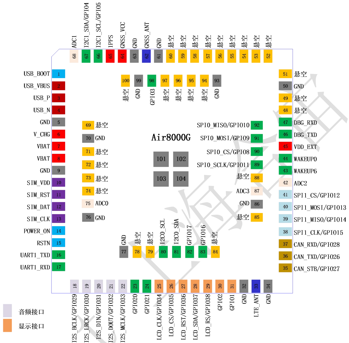
图表 4: Air8000G 管脚排列图（正视图）
