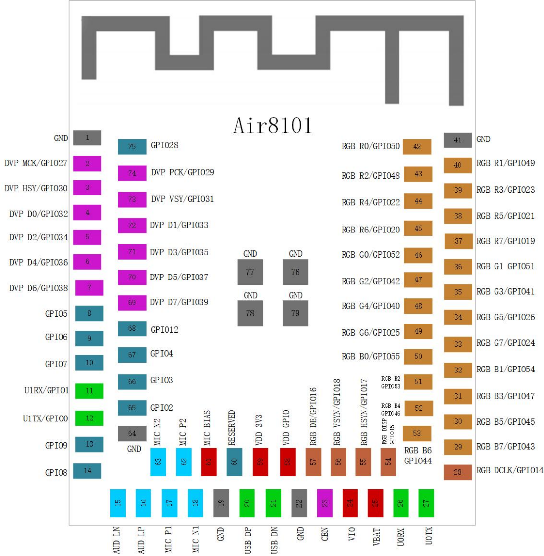
管脚透视图
