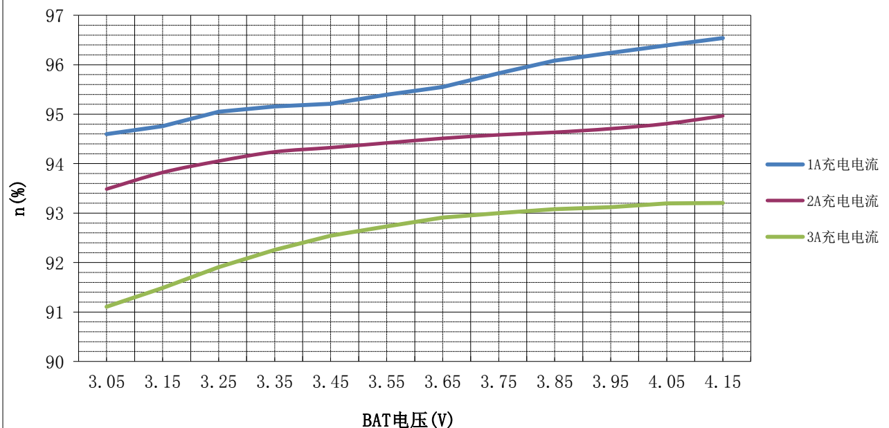
IP2312U充电效率曲线 VIN=5V
