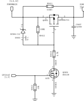
UART11转485接口/供电
