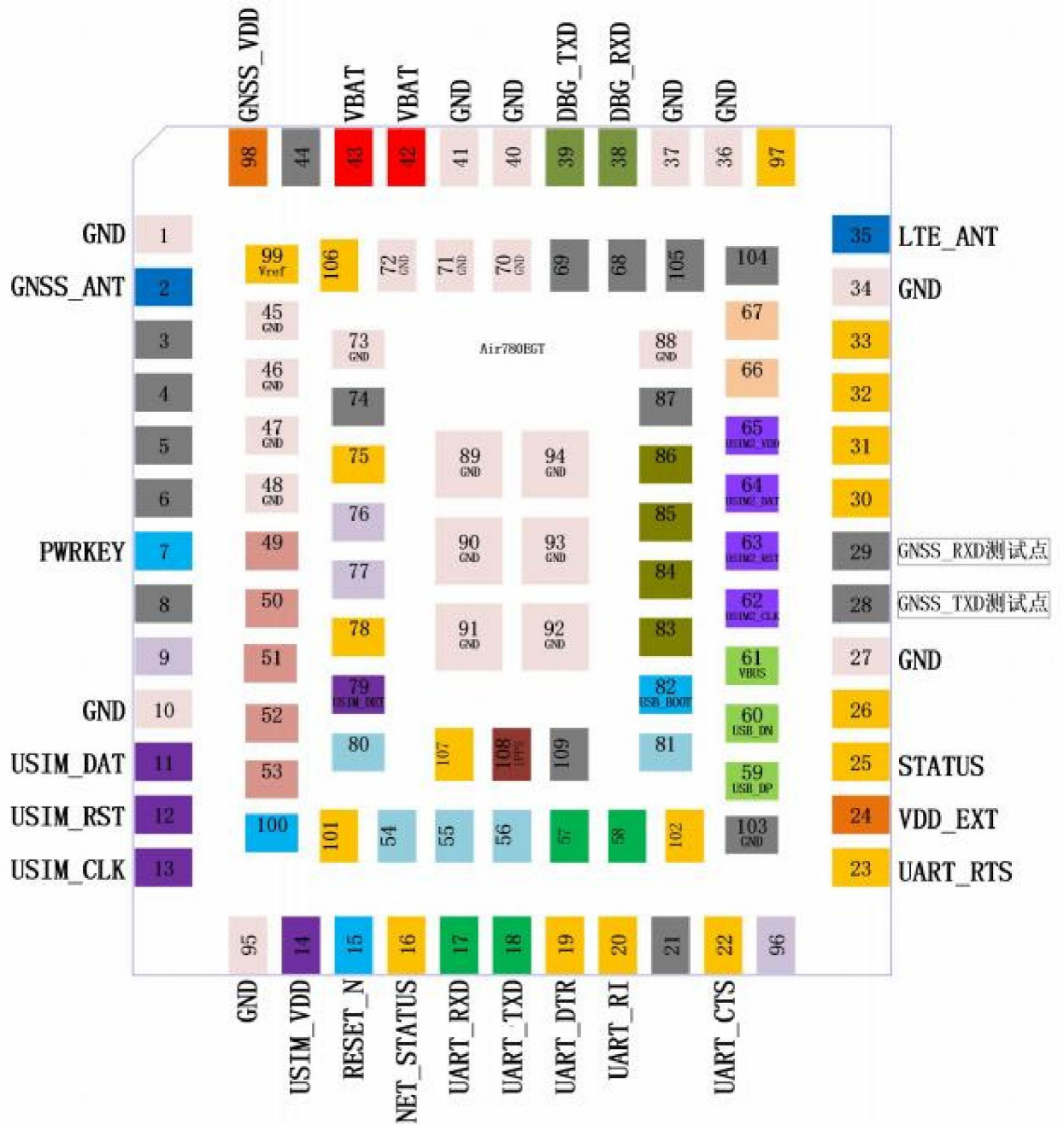
管脚透视图
