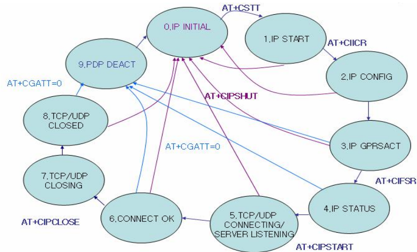
图 1：单链接时的状态机
